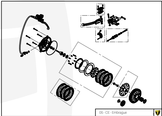
05 - CE - Embrague
