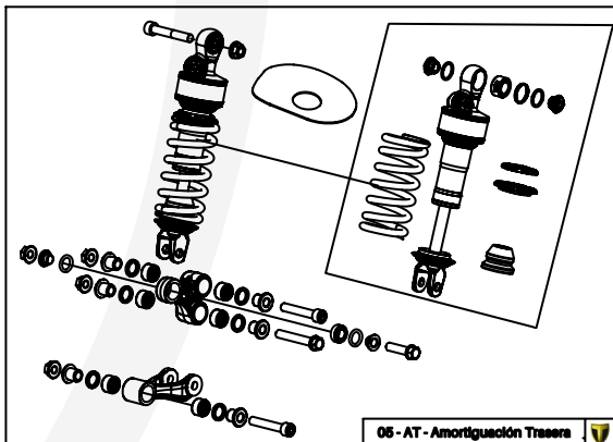
06 - AT - Amortiguación Trasera
