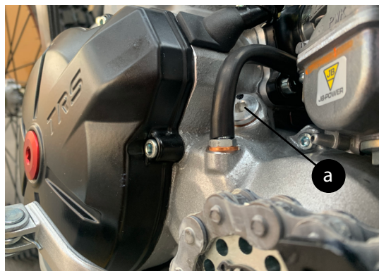
a): Tapón llenado aceite, en la parte superior del cárter.
