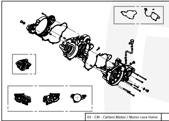
03 - CM - Cárters Motor / Motor case Halve
