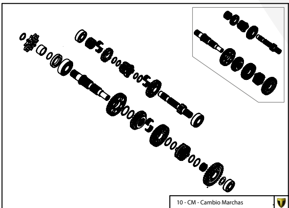
10 - CM - Cambio Marchas
