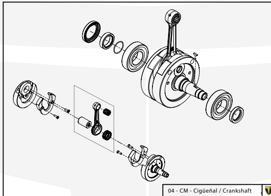
04 - CM - Cigüeñal / Crankshaft
