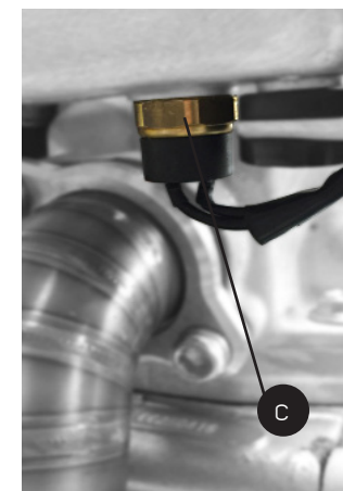
b) Termocontacto situado en la parte inferior del radiador.
