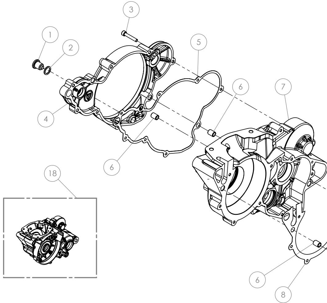
Graphic Engine Longer Bolts - Gráfico Longitud Tornillos
